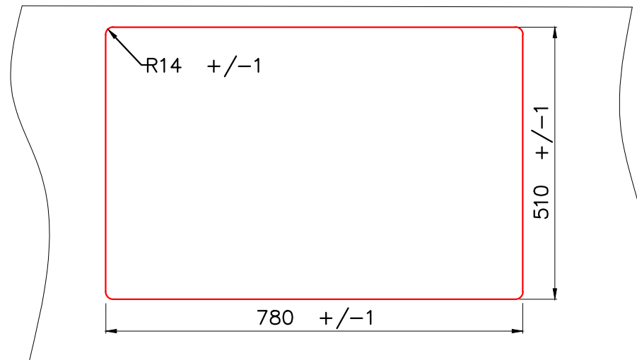
Врезной монтаж мойки (I)
